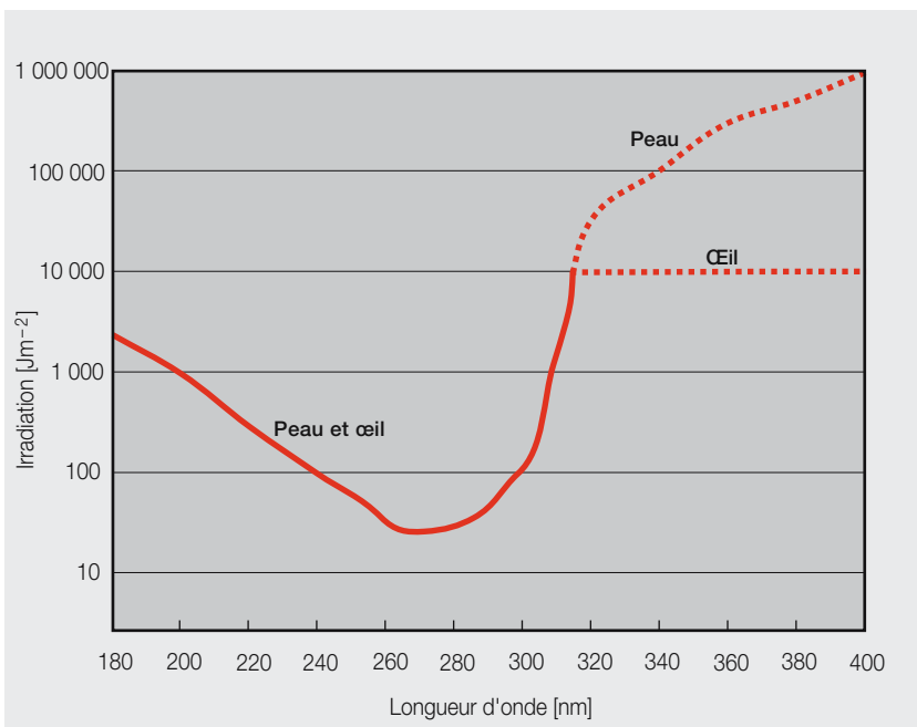
Figure 1: Irradiation UV maximale admissible pour une durée de 8 heures (journée de travail). Représentation graphique des valeurs limites du tableau 2 (page 142).
